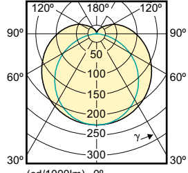
(cd/1000lm) 0° — 0-180° — 90-270°
